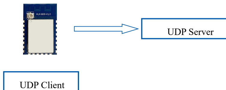
图 12 UDP Client
