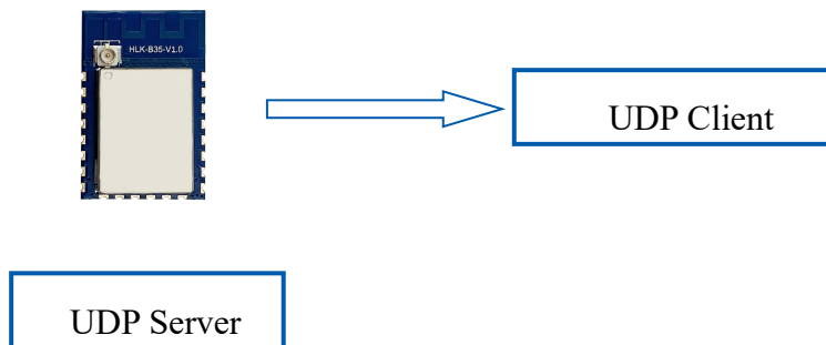
图 11 UDP Server
